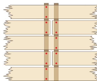
vhodný způsob uložení kolmých styků terasových palubek
