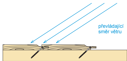
Vertikální orientace fasádních palubek s perem a drážkou, pero musí směřovat proti převládajícímu směru větru. Neviditelné připojení vruty RAPITEC® BSP do palubek a lišt
