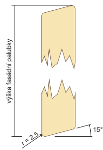
Úprava konců fasádních palubek při vertikální orientaci
