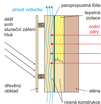
Schéma konstrukce opláštěné vertikálně orientovaným obkladem. Kotevní prvky prochází přes nosníky.
