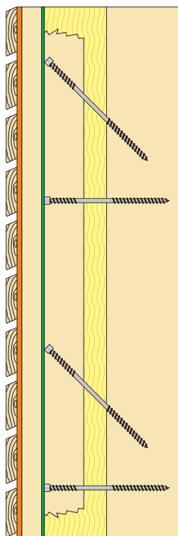
Ukotvení vruty Toproof
