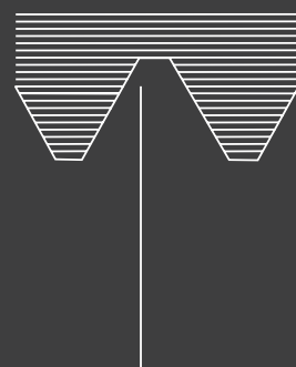
Fibre structure of thread cutting Andamento delle fibre per filettatura tagliata
