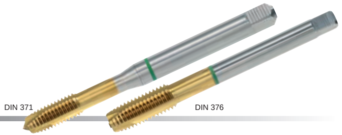
DIN 371/376 Form B HSSE-PM-TIN Tol. ISO2/6H
