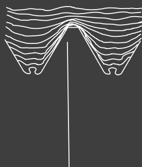
Fibre structure of thread forming Andamento delle fibre per filettatura rullata
